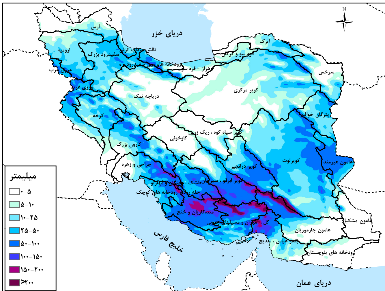
شکل ۱- پیش‌بینی بارش تجمعی از بامداد روز شنبه مورخ ۲۵ دی تا انتهای روز سه‌شنبه مورخ ۲۸ دی ماه ۱۴۰۰ (بر اساس نتایج مدل WRF با زمان پایه ساعت ۳:۳۰ روز شنبه مورخ ۲۵ دی ۱۴۰۰)
